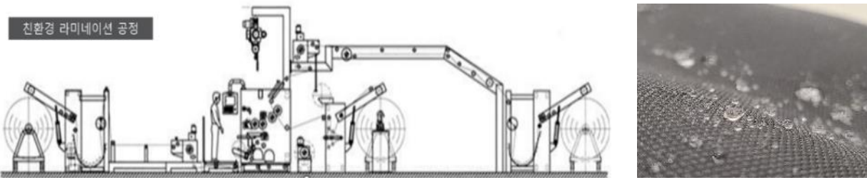
불소가 포함 안된 탄화수소, 아크릴, 실리콘계 소재를 사용한 발수제 및 투습 방수원단 개발
